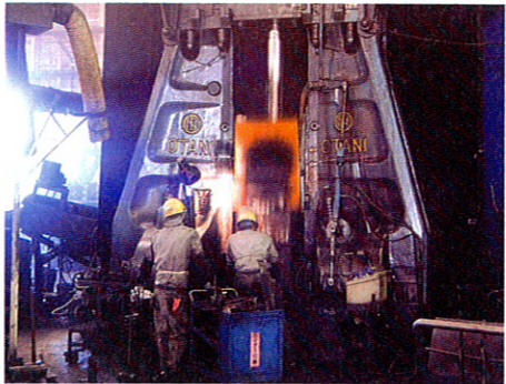
3Tonエアドロップハンマー
