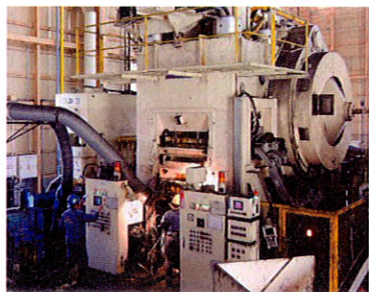
2500Tonウェッジプレス
